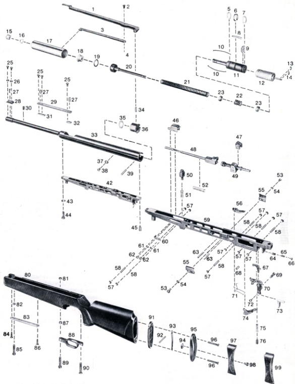
Admetus LG 250. Für die Benennung der abgebildeten Teile, siehe Literatur des Herstellers
